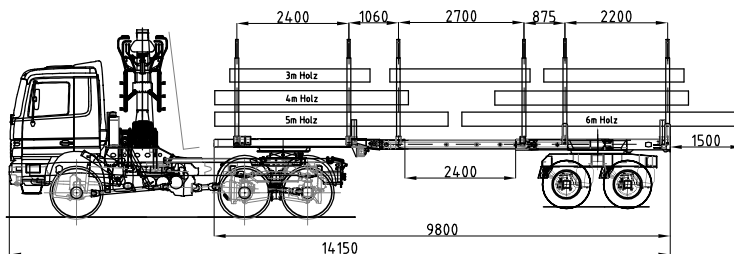
Rahmen in Ladestellung
