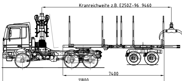
Rahmen in Ladestellung
